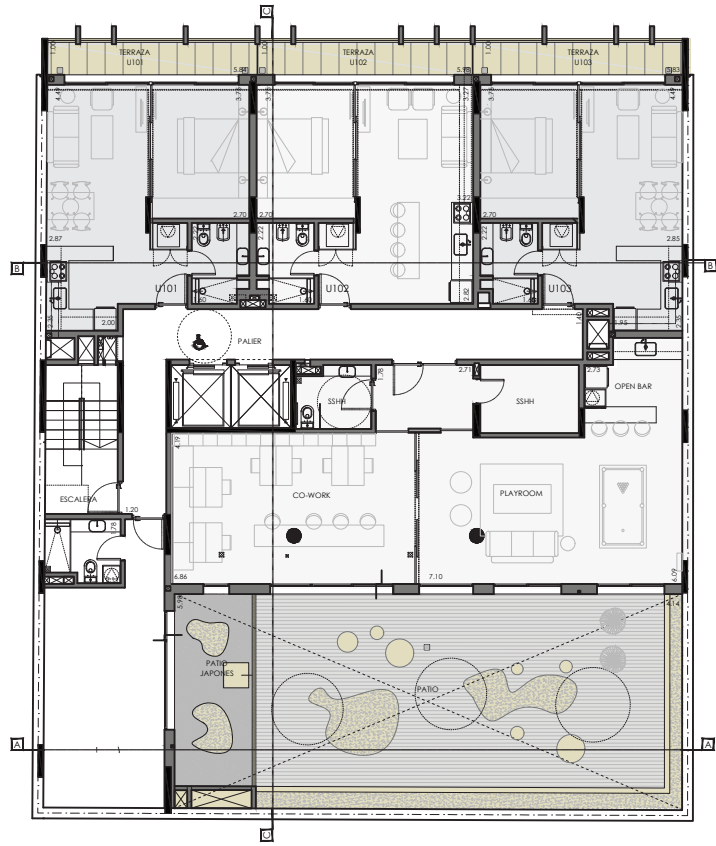
PLANTA 1º
