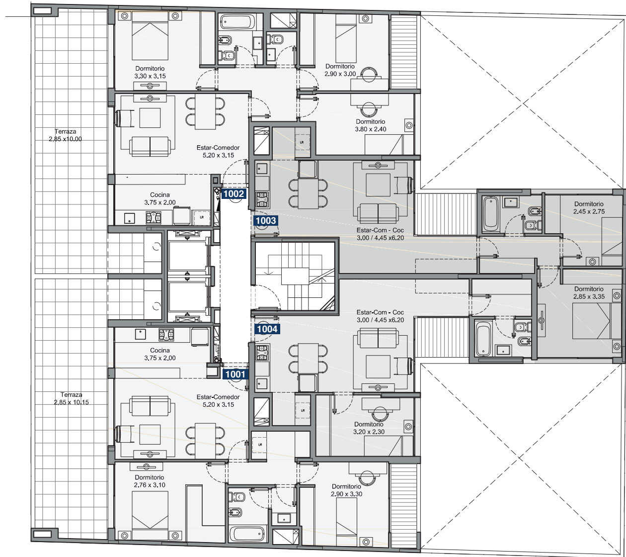
PLANTA PISO 10º GALIBO
