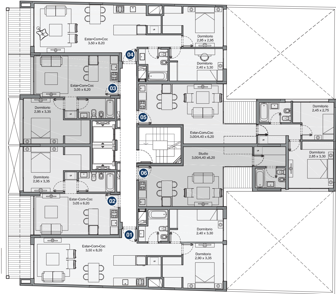
PLANTA PISO 2º a 9º
