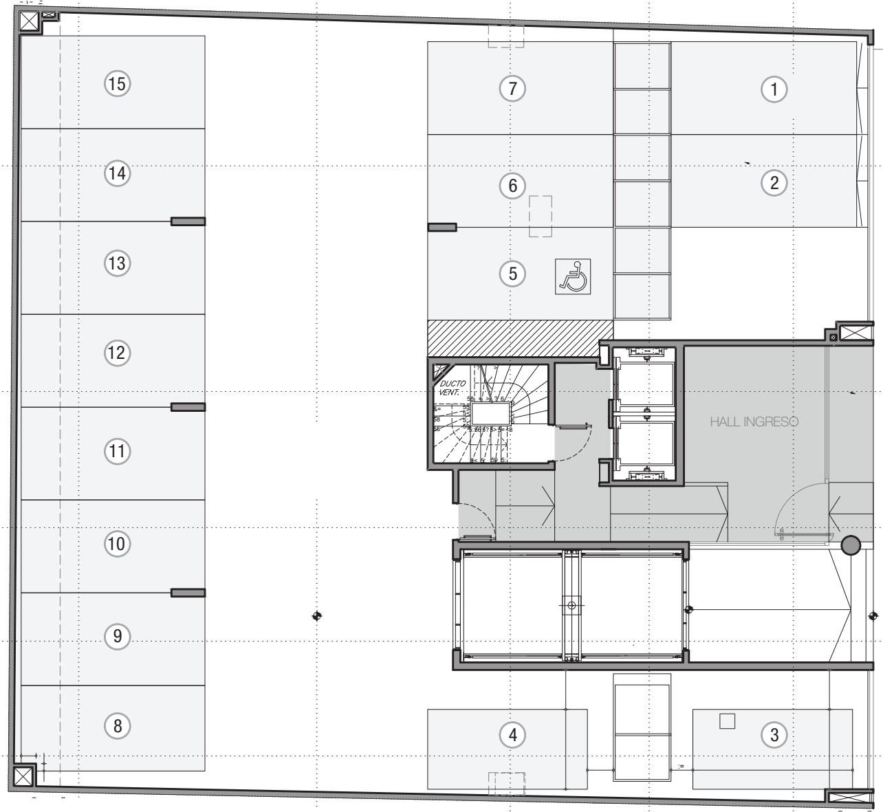
PLANTA BAJA / HALL / COCHERAS
